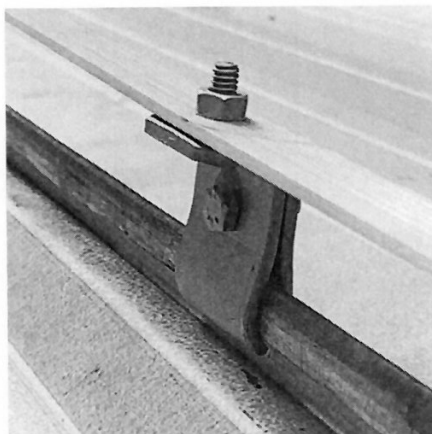
Figura 1 - CONECTOR PARA TELHA ZIPADA
